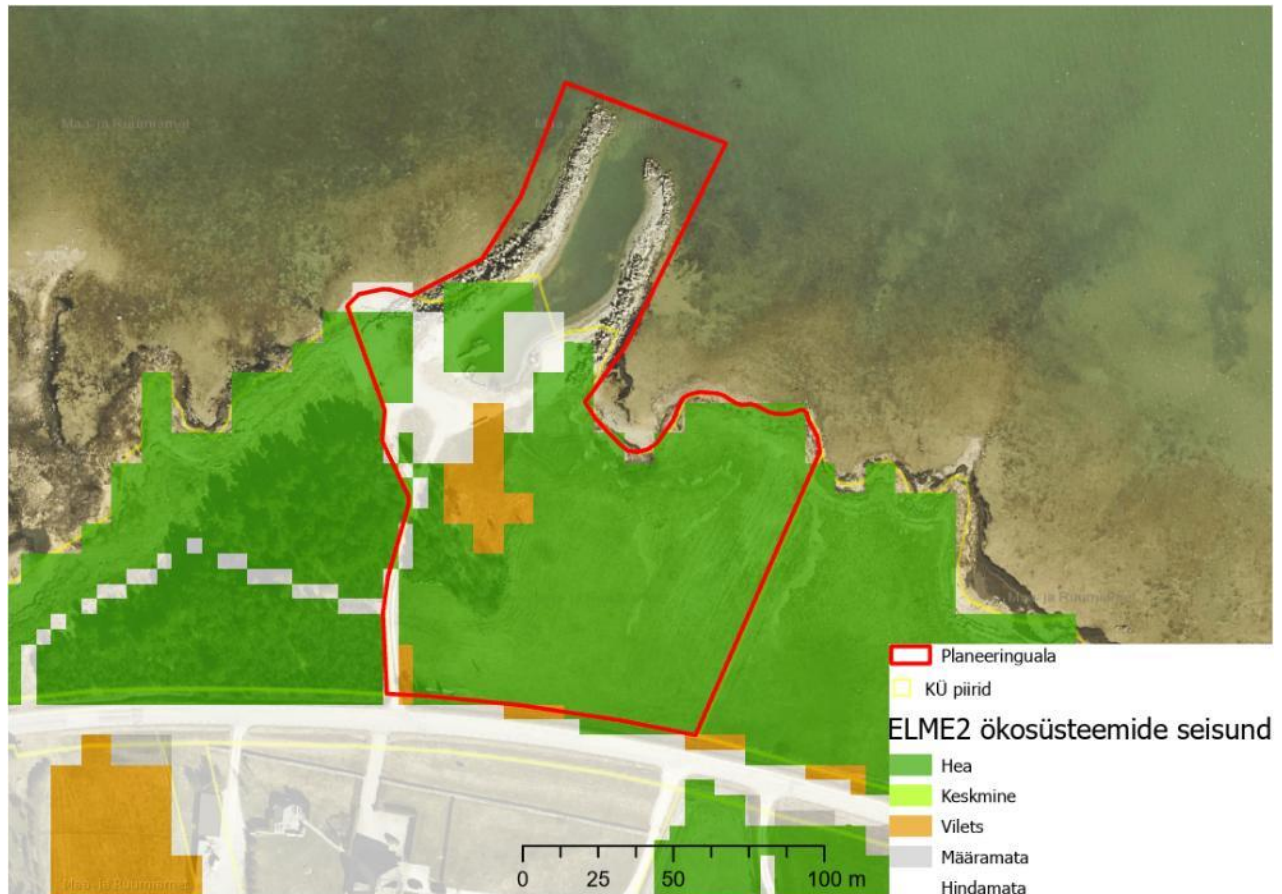
Joonis 7. Ökosüsteemide seisund planeeringualal. Alus: ELME2 projekt, Keskkonnaagentuur.
